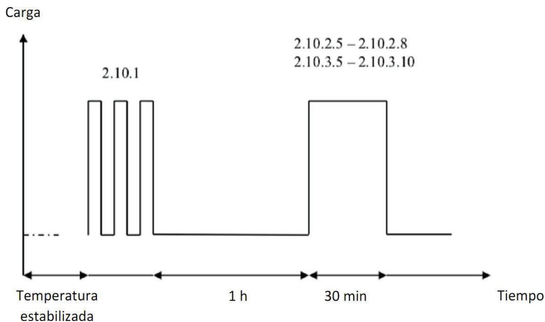
Figura 2 Secuencia de ensayo recomendada para cada temperatura de ensayo, para los ensayos de retorno a cero (DR) y de creep cuando los ensayos se realizan en una máquina de ensayo diferente a la usada para los ensayos de carga.
